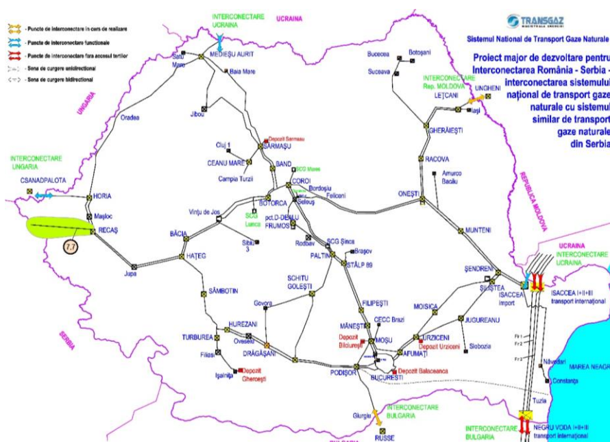
Figura 16 - Interconectarea SNT cu Serbia pe direcția Receaș–Mokrin
