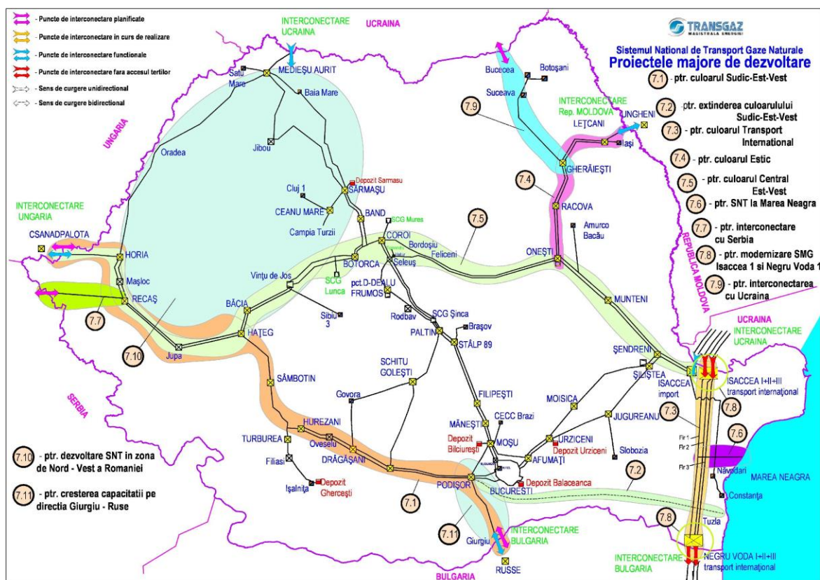
Figura 7 - Harta proiectelor majore din SNT
