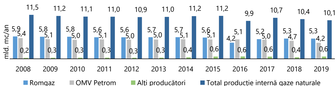
Grafic 11 – Producția internă de gaze naturale în funcție de principalii producători în perioada 2008-2019 (mld mc/an)
