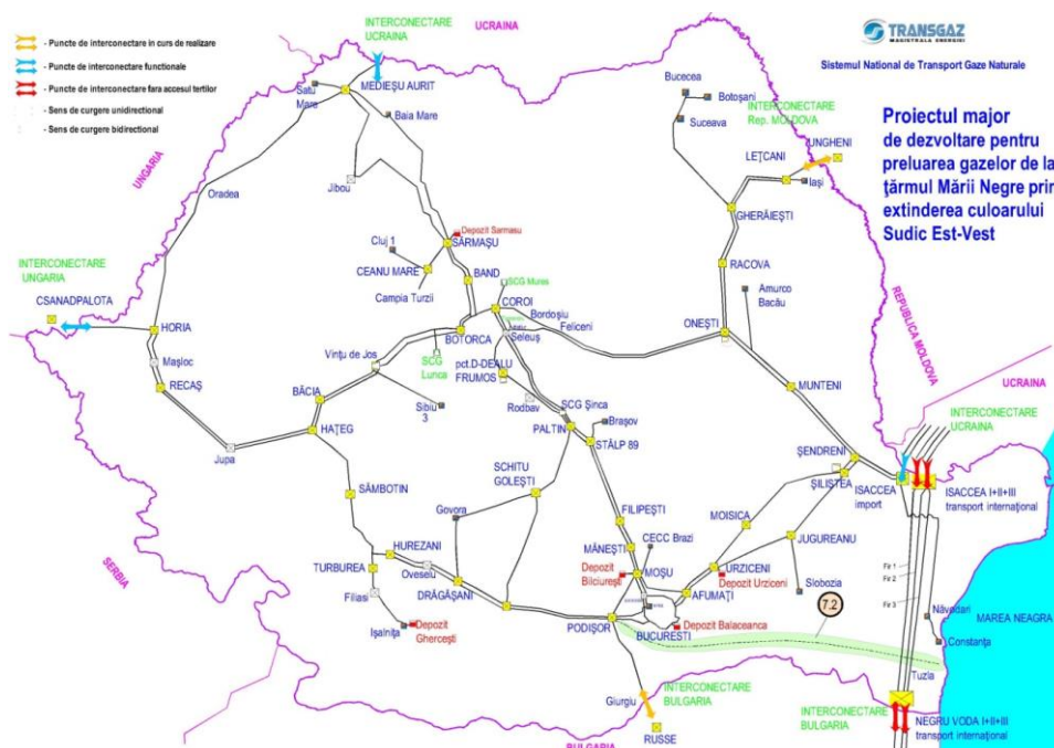
Figura 11 - Harta proiectului major de dezvoltare pentru preluarea gazelor de la țărmul Mării Negre prin extinderea culoarului Sudic Est-Vest
