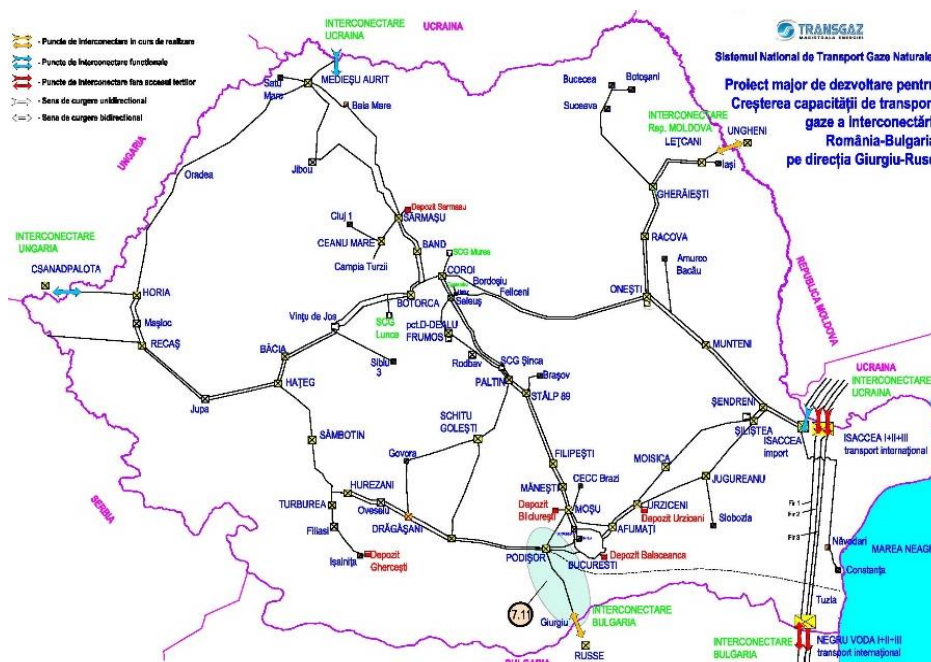
Figura 20- Creșterea capacității de transport gaze naturale a interconectării România-Bulgaria pe direcția Giurgiu-Ruse
