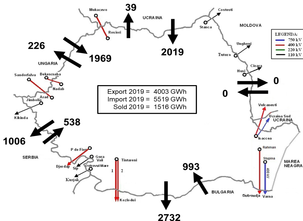
Fig. 5.2.4 – Schimburile de energie realizate pe granițe în anul 2019
