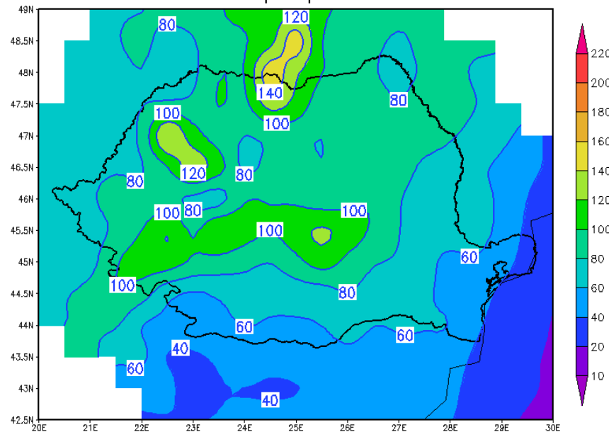
Media multianuală a precipitațiilor cumulate lunie
