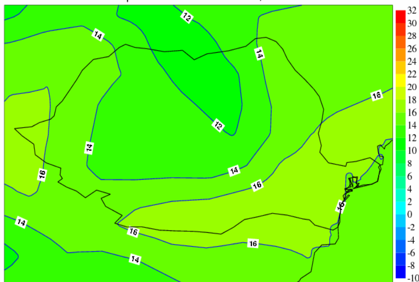
Temperatura Medie la 2 m Mai, 2016
