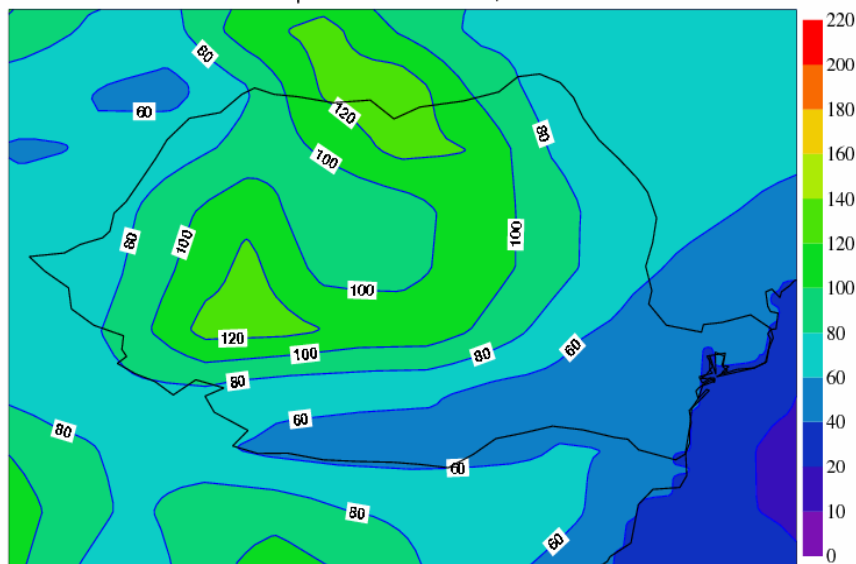
Precipitații cumulate Mai, 2016
