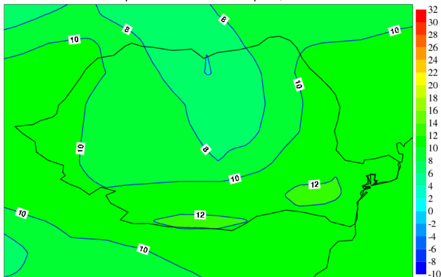
Temperatura Medie la 2 m Aprilie, 2016
