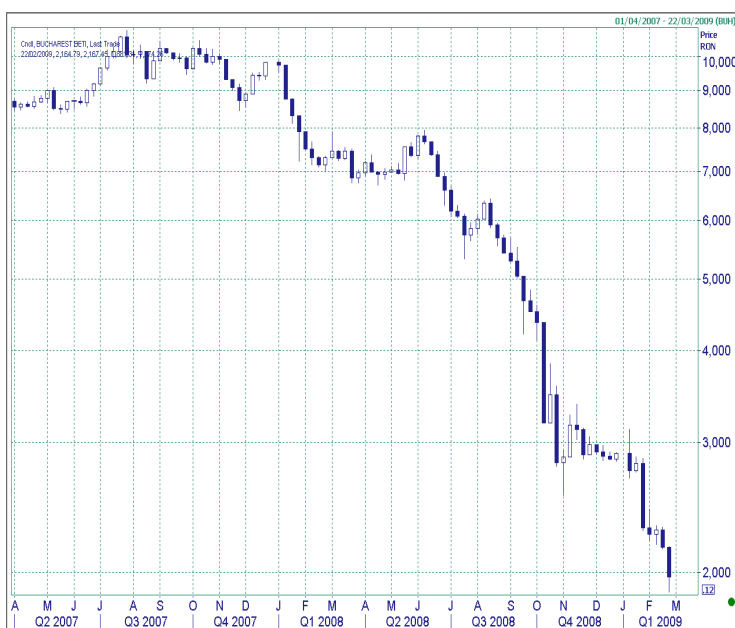
Indicele BET
