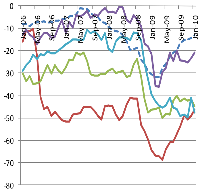
Încrederea consumatorilor
