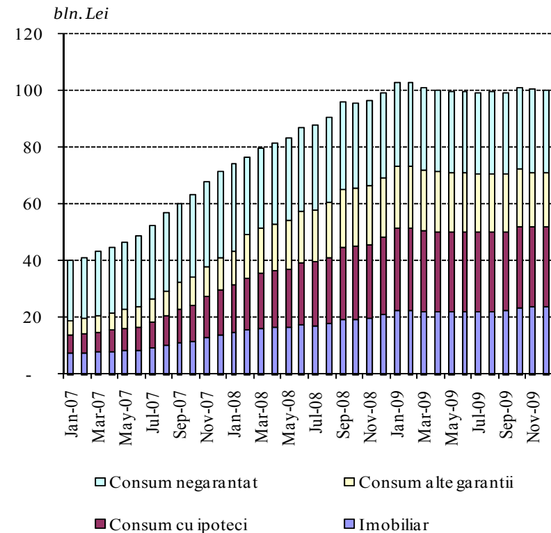
Credite - populație
