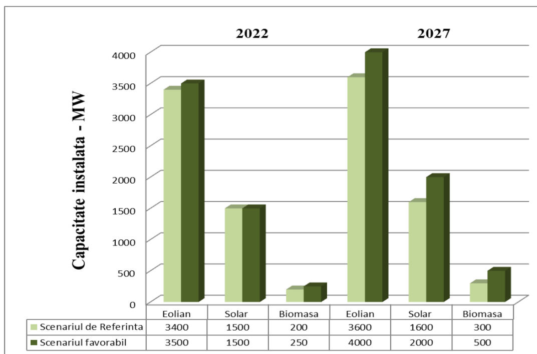
Fig.9.4.2 Evoluția capacităților de producere
