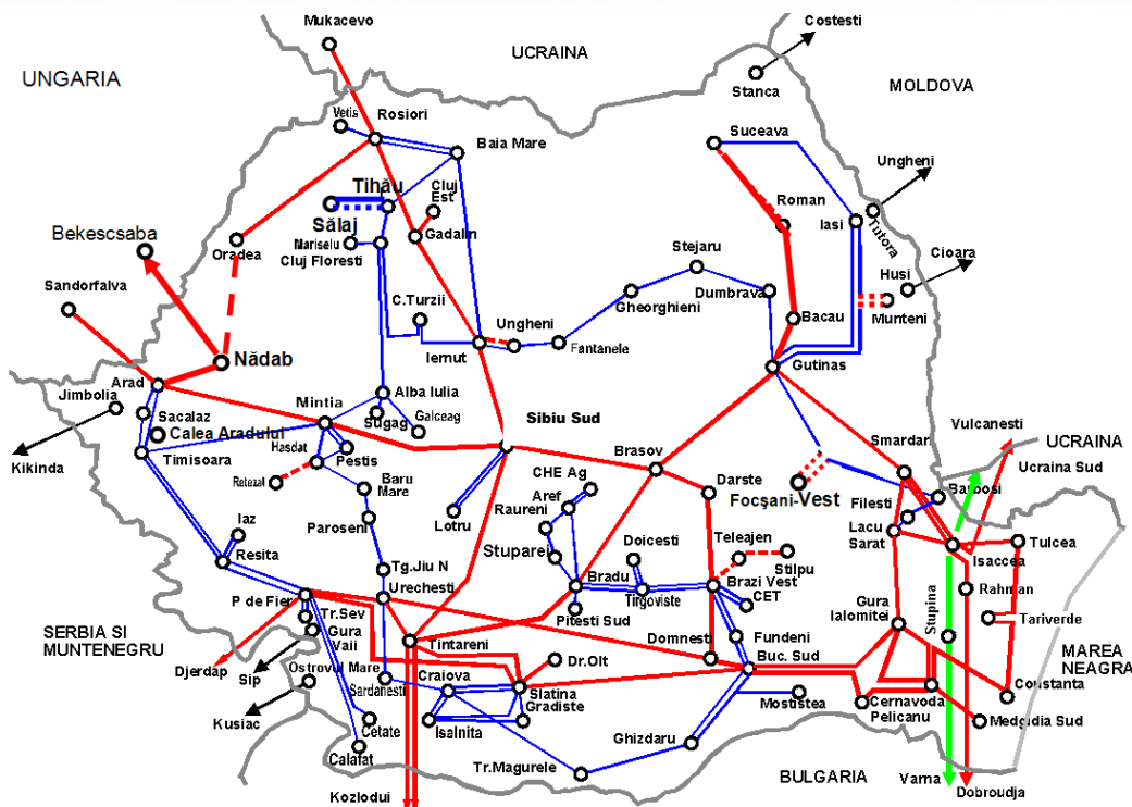
Fig. 5.3 Rețeaua Electrică de Transport – octombrie 2017
