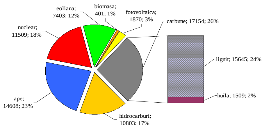
Structura pe resurse primare [GWh;%] a producției brute de energie electrică în anul 2017
