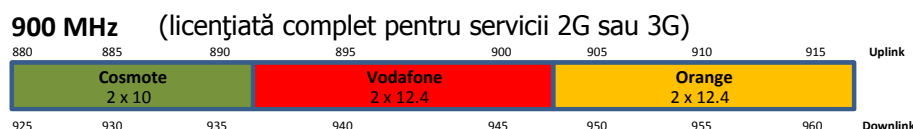
Figura 2 – Poziționarea alocărilor actuale în banda de 900 MHz
