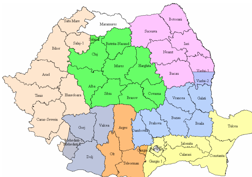
Figura 9 – Definierea celor 7 zone în aria de dezvoltare backhaul RONET
